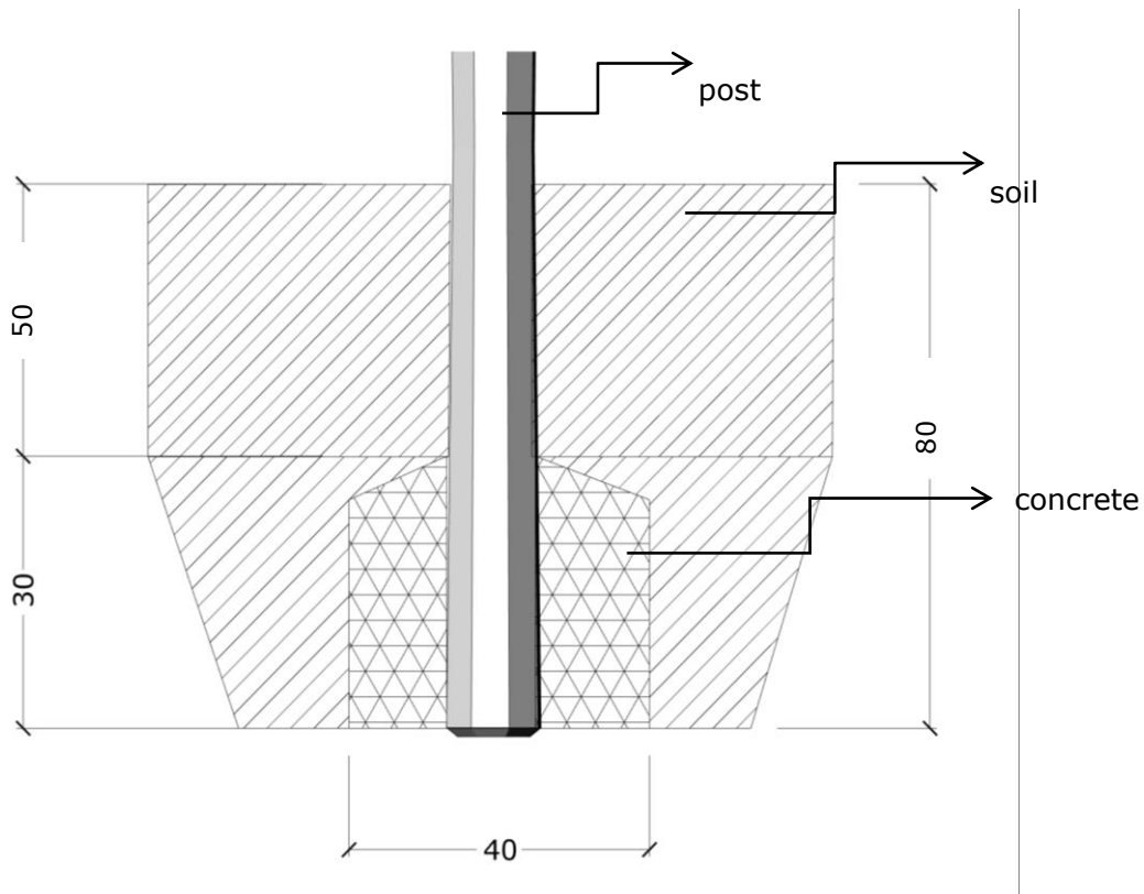
Foundation, FD F1
