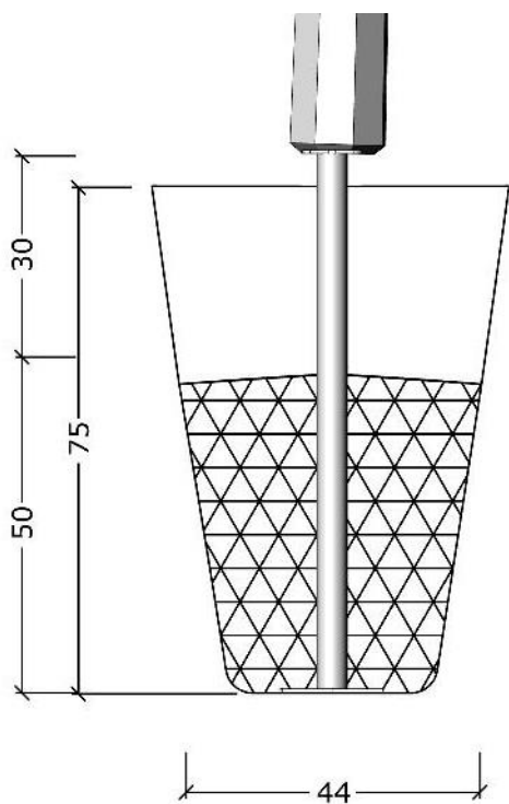
Fundering "benzinsrander"
