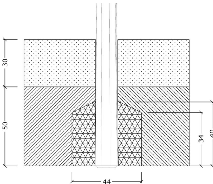
Fundering Stolper til tag
