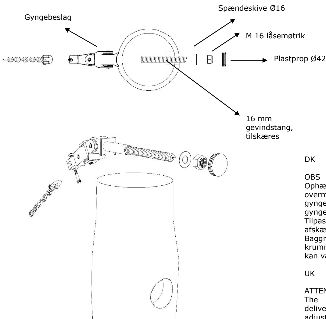
Montageprincip MP 06
